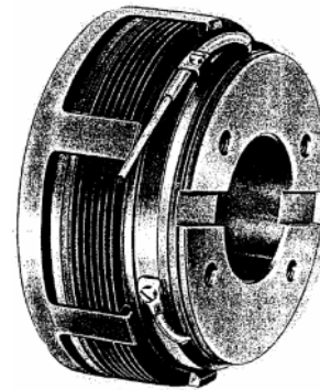
Kupplungsaufbau - selbstnachstellende Lamellenkupplungen (können auch nass eingesetzt werden) Ausführung EKN, EKN... B
