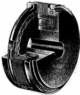
Kupplungsaufbau - selbstnachstellende Lamellenkupplungen (können auch nass eingesetzt werden) Ausführung EKN, EKN... B
