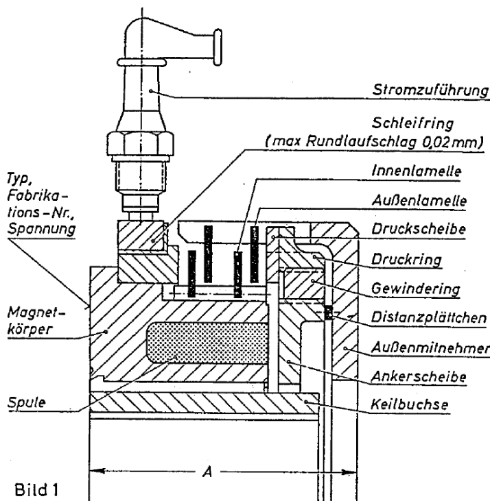
Kupplungsaufbau - selbstnachstellende Lamellenkupplungen (können auch nass eingesetzt werden) Ausführung EKN, EKN... B
